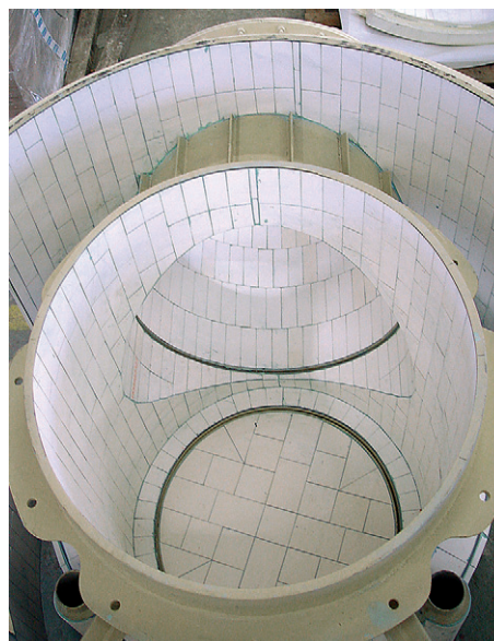
Kalocer-vuorattu luokitin.
